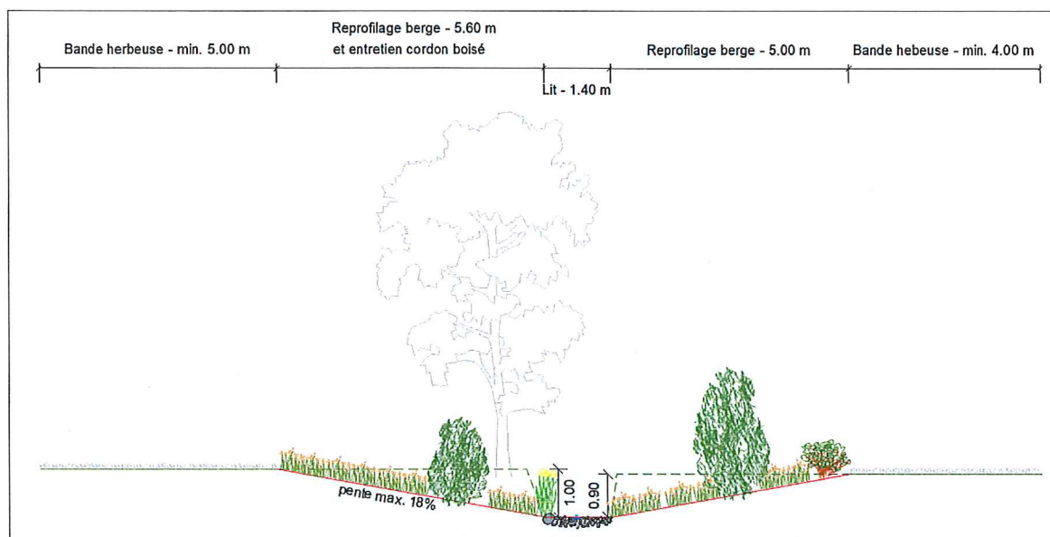
Exemple de reprofilage des berges proposé
